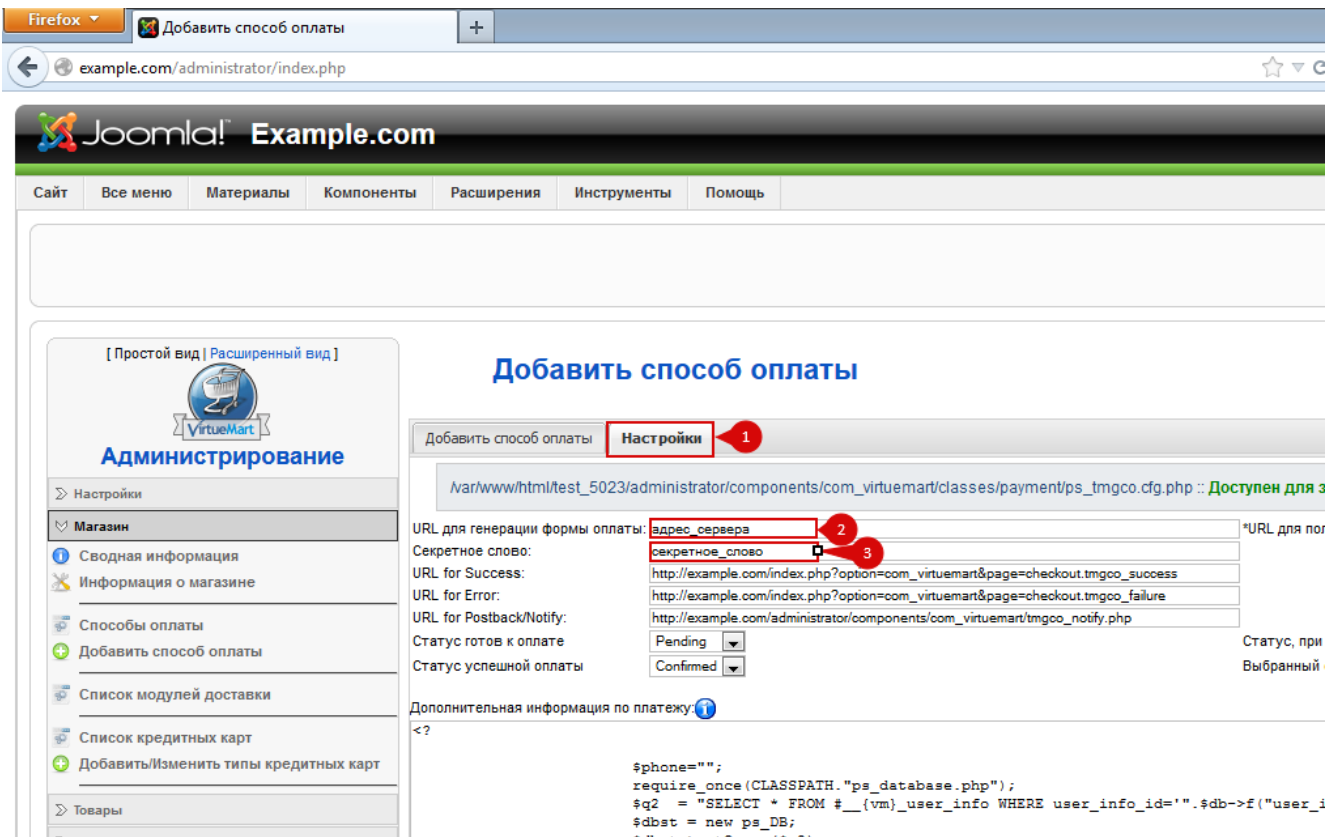
Рисунок 4. Настройка модуля
